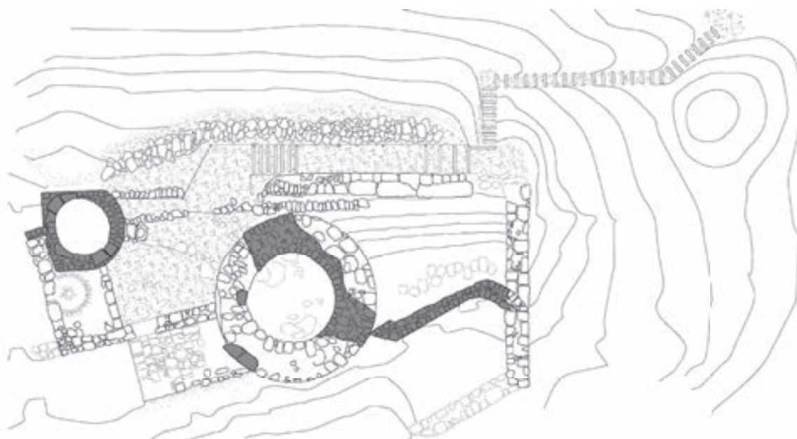
PLANTA TRAS REHABILITACIÓN
