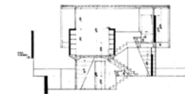
figura 10 Sección transversal de la casa Rubens de Mendonça, conocida como casa dos Triângulos (São Paulo, 1958). Fuente: Acervo João Batista Vilanova Artigas
