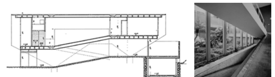
figura 19 Sección longitudinal de la casa Tacques Bittencourt (São Paulo, 1966). Las rampas discurren perpendicularmente a la calle y alrededor del patio, siguiendo una procesión ascendente. Fuente: Acervo João Batista Vilanova Artigas.
