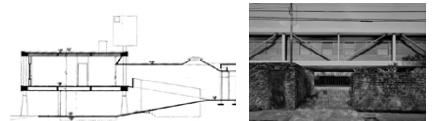
figura 17 Sección transversal de la casa Mendes André (São Paulo, 1966). Obsérvese la ligera elevación respecto al plano de calle. Fuente: Acervo João Batista Vilanova Artigas
