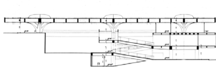
figura 23 Sección longitudinal de la estación de autobuses de Jaú (1973). Acervo João Batista Vilanova Artigas
