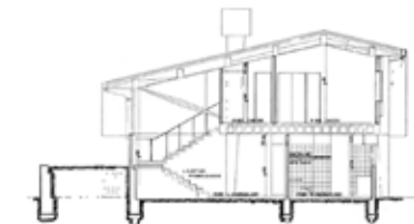
figura 7 Sección transversal de la casa Baeta (São Paulo, 1956). Fuente: Acervo João Batista Vilanova Artigas
