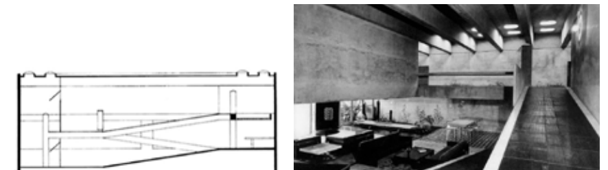
figura 14 Secciones de la casa Telmo Porto (São Paulo, 1968). Acervo João Batista Vilanova Artigas
