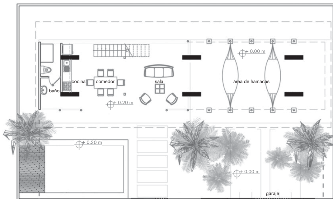
PLANTA BAJA
